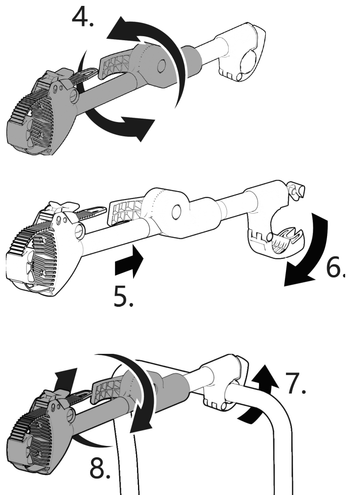
Figure 4 : Montage sur l'étrier en U
