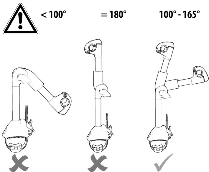
Figure 2 : Déploiement du support de cadre
